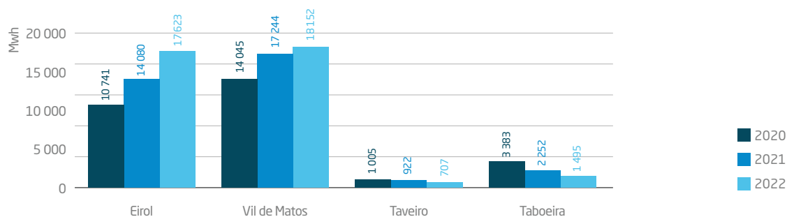
Figura 11. Energia elétrica injetada na rede nos diferentes sistemas da ERSUC triénio 2020-2022
