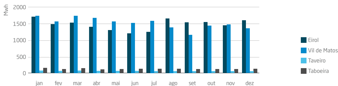
Figura 12. Produção de Energia MWh 2022 por instalação
